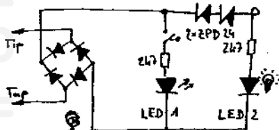
BILD 1: Prüfstift (Schaltung)
