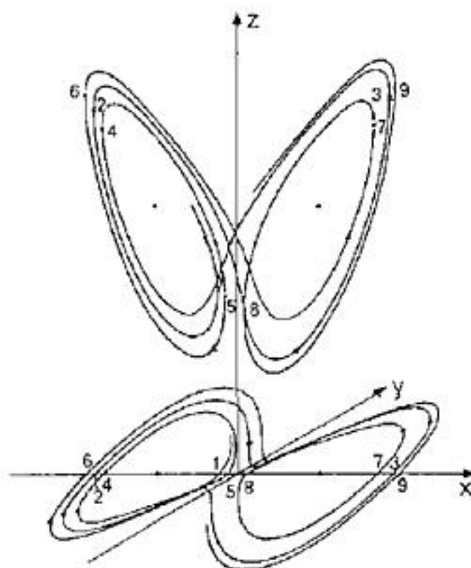
Abb. 12.2. Obere Hälfte: Trajektorien in der Projektion auf die (X, Z)-Ebene. Untere Hälfte: Trajektorien in der Projektion auf die (X, Y)-Ebene. Die Punkte gehören zu stationären Lösungen. Nach M. Lücke
